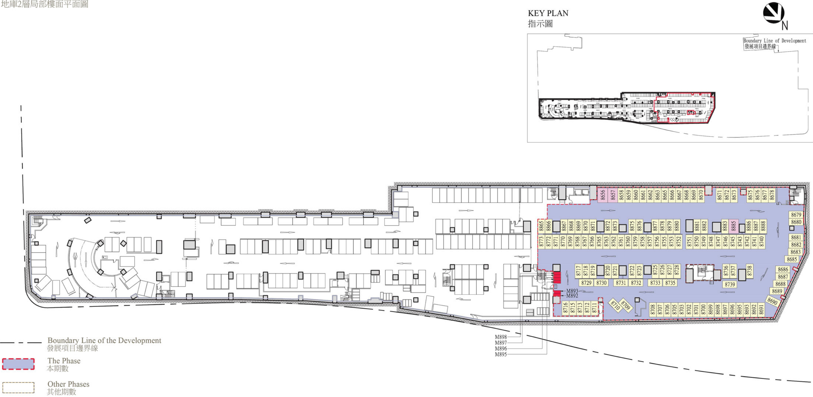
B2/F Part Floor Plan 地庫2層局部樓面平面圖
